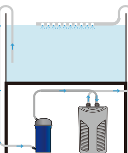
① 外部フィルターとの接続
